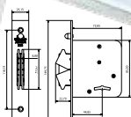
CÓD. 10139 DOBLE GANCHO DESCRIP. CERROJO 525 MATERIAL H. BIC. PLACAS 4 AC. GALV. PASADOR DOBLE GANCHO
