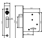
CÓD. 10130 JUNIOR DESCRIP. CERROJO 500R MATERIAL H. BIC. PLACAS 4 AC. GALV. PASADOR RECTANGULAR
